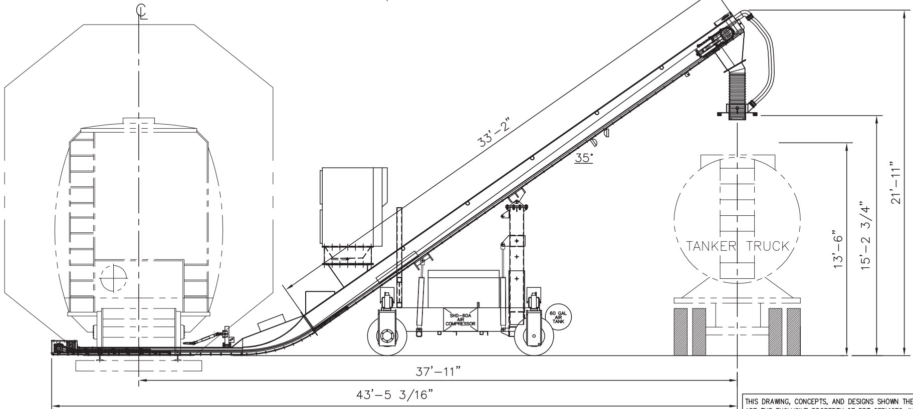
ELEVATION
